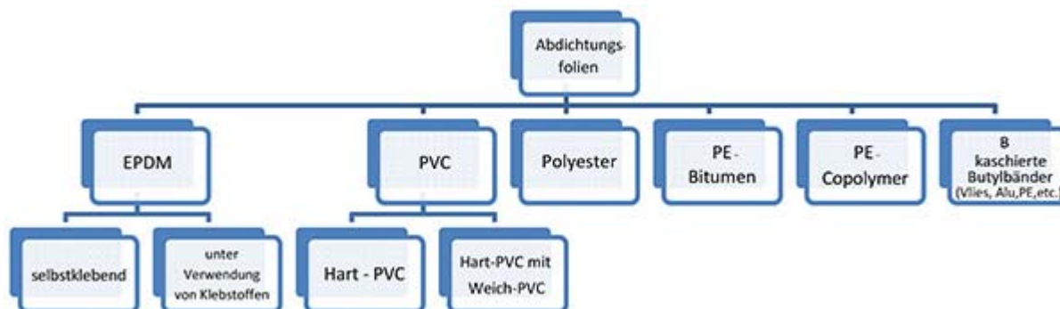
Abbildung 11: Einteilung der Abdichtungsfolien
