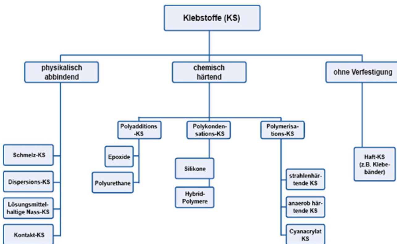
Abbildung 12: Übersicht der Klebstoffe
